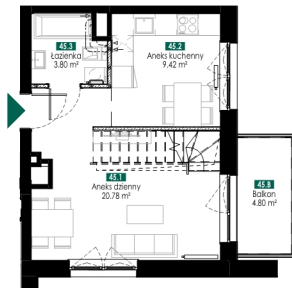
poziom dolny
