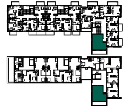
RZUT KONDYGNACJI IV PIĘTRO + ANTRESOLA
