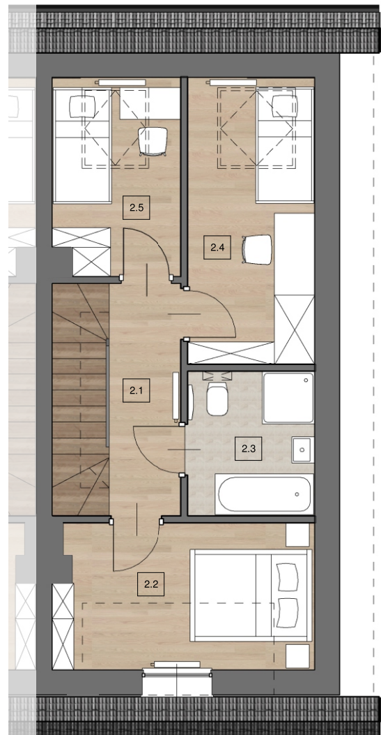
RZUT PIĘTRA
